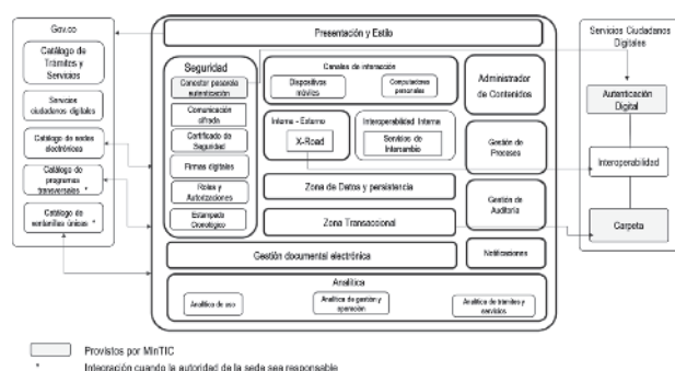
Figura 1. Arquitectura de referencia de una sede electrónica
